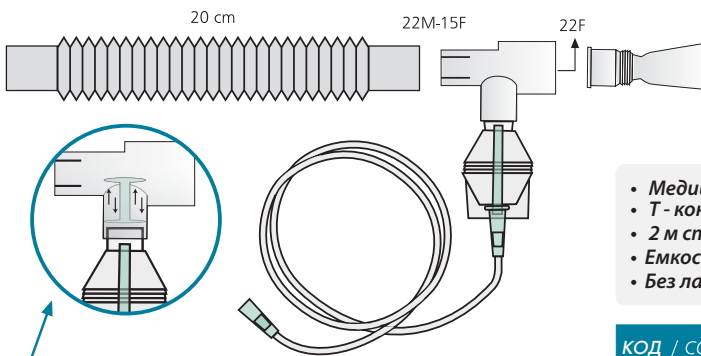
130 205 T-коннектор с клапаном T part and valve
